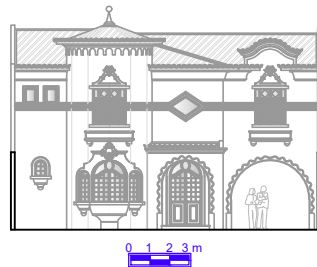
Elevation 01
